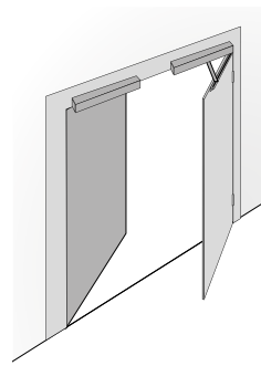
Kozijndorpel-installatie (2 deurvleugels met tweerichtingsverkeer) Tegengestelde werking van twee aandrijvingen
