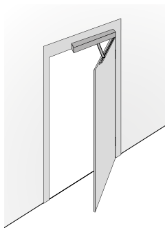
Kozijndorpel-installatie (1 deurvleugel) Standaardarm DIN-links of -rechts trekkend
