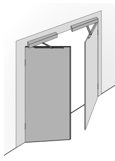
Kozijndorpel-installatie (2 deurvleugels, Master-Slave) Twee elektrisch gekoppelde aandrijvingen met standaardarm trekkend
