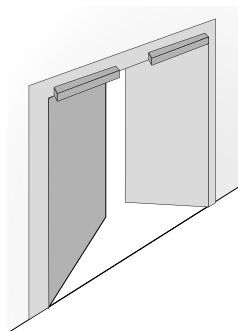
Kozijndorpel-installatie (2 deurvleugels, Master-Slave) Twee elektrisch gekoppelde aandrijvingen met standaardarm duwend
